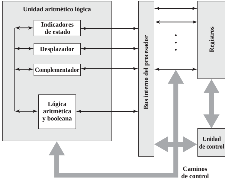
Figura 12.2. Estructura interna del procesador.
