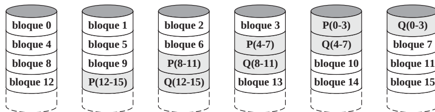
(d) RAID 6 (redundancia doble)
